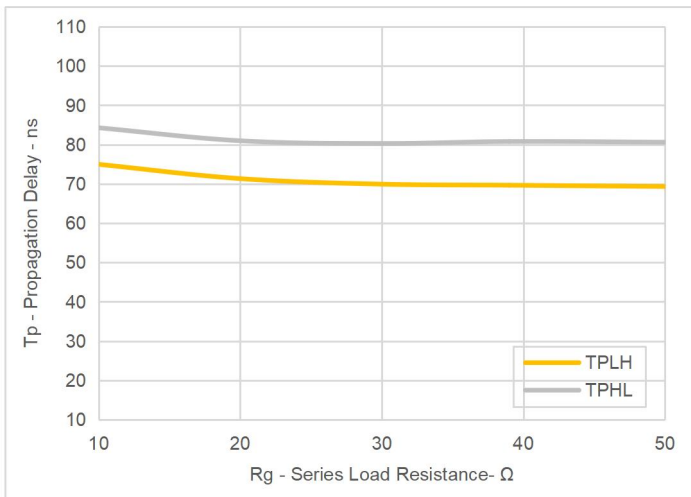
图例 11-传输延时与负载电阻曲线图 Fig.11 Propagation Delays vs. Rg
