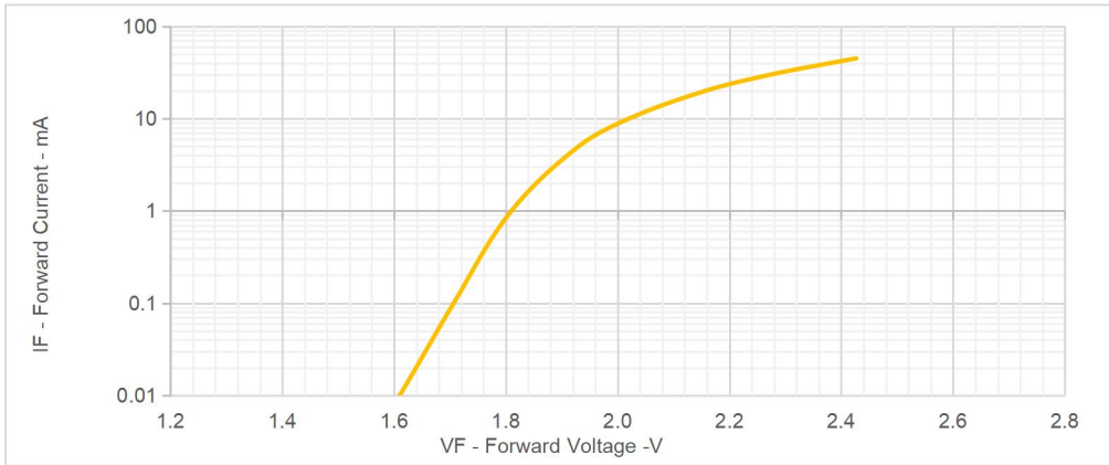
图例 13-正向电流与正向电压曲线图
