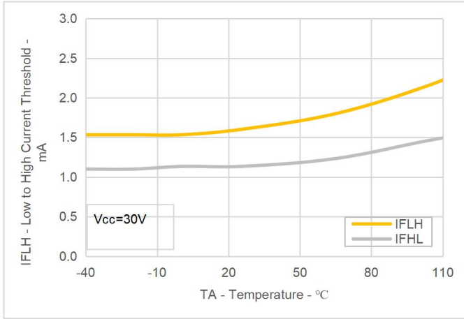
图例 7-阈值电流从低到高与工作温度曲线图 Fig.7 IFLH vs. Temperature
